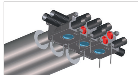
Luftverteiler MF-VK90-7 kombiniert mit herkömmlichen Schalldämpfern
