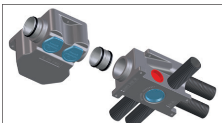
Schalldämpfer-Box mit Luftverteiler MF-VK90-7 mit max. 7 Anschlussoptionen DN 90 für Flexrohre
