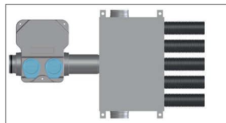
Schalldämpfer-Box mit Luftverteiler aus Stahlblech mit 5 Anschlussoptionen DN 90 für Flexrohre
