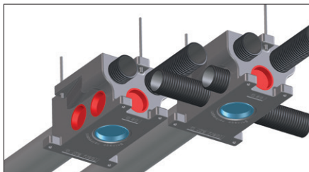
Dank versetzter Anschlüsse lassen sich die Flexrohre DN 90 problemlos aneinander vorbei führen
