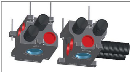
Luftverteiler MF-VK90-7 um 180° gedreht passen exakt aneinander
